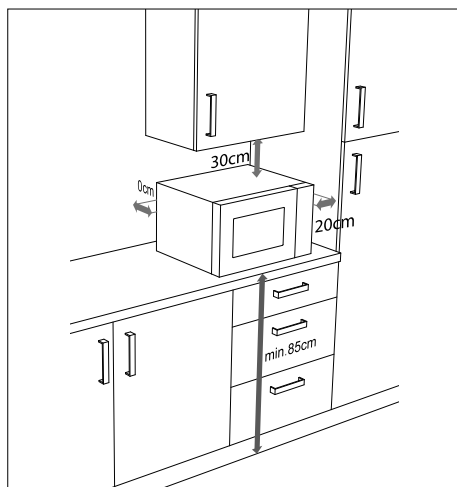
Fig. 3 – Distancias del aparato
