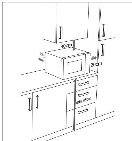
Abb. 3 – Geräteabstand
