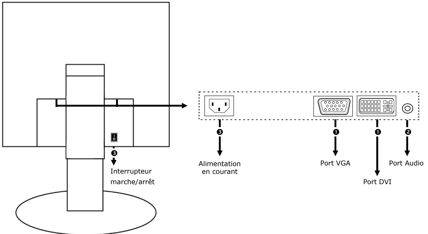
(Ill.: Ports à l'arrière)
